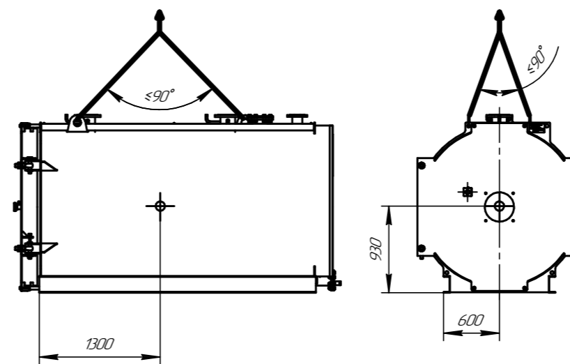
Схема строповки
